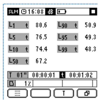
Pantalla estadística: muestra el valor de los percentiles
