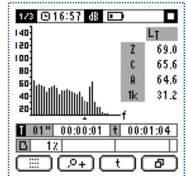
Pantalla gráfica: muestra en tiempo real el espectro medido
