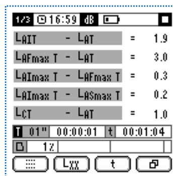
Pantalla avanzada: Muestra funciones acústicas especiales
