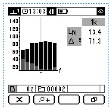
Pantalla gráfica de niveles de ruido: muestra su espectro
