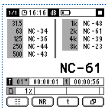
Pantalla curvas: Evalúa el espectro según las curvas NC y NR
