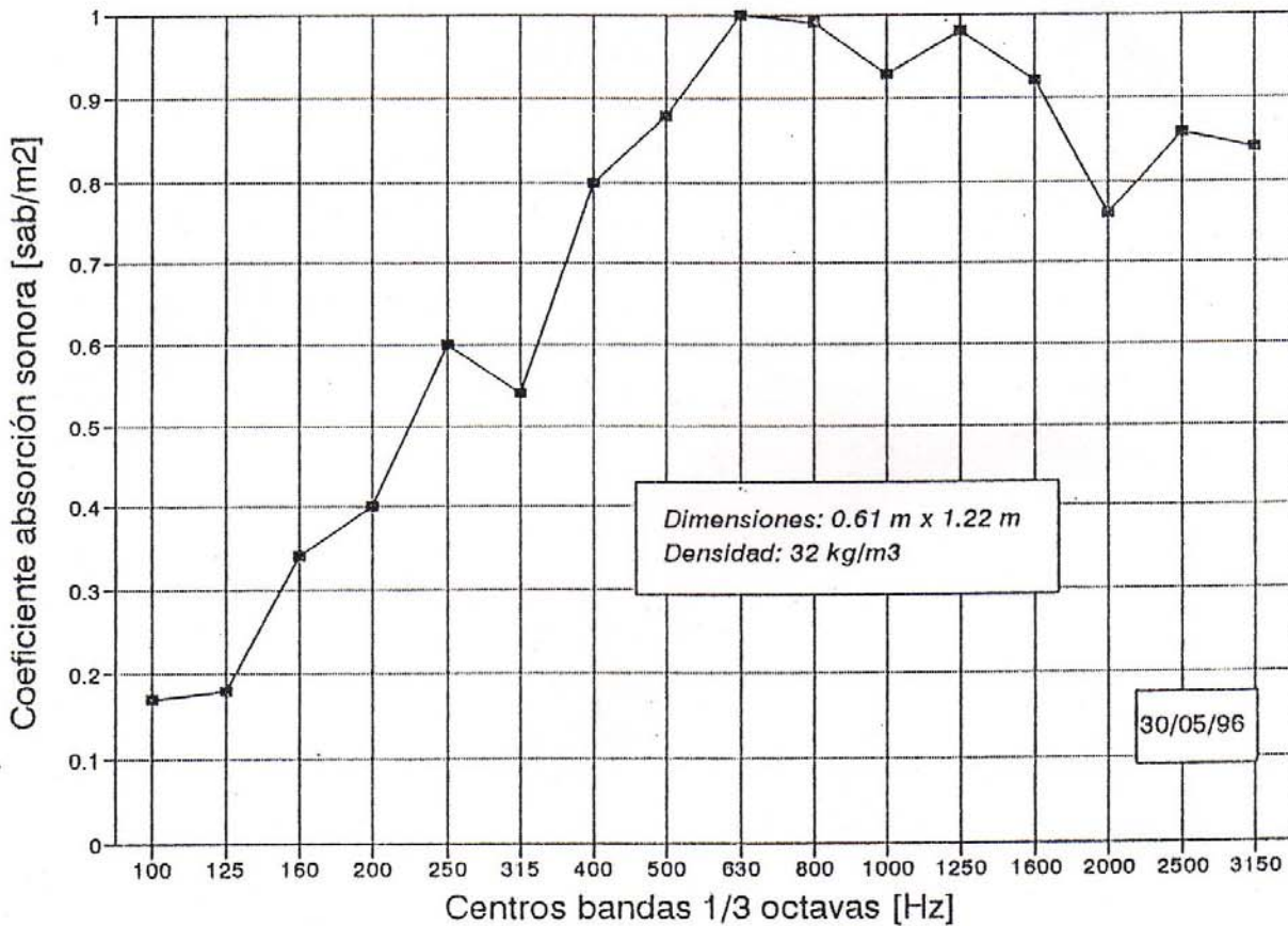
Figura 1: Placas FONAC PRO, e: 75 mm Laboratorio CINAC-INTI, norma IRAM 4065
