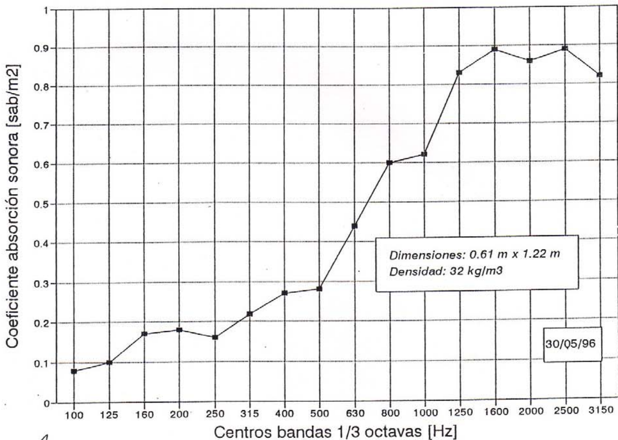
Figura 1: Placas FONAC PRO, e: 20 mm Laboratorio CINAC-INTI, norma IRAM 4065
