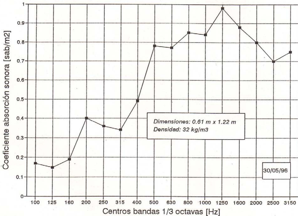
Figura 1: Placas FONAC PRO, e: 50 mm Laboratorio CINAC-INTI, norma IRAM 4065
