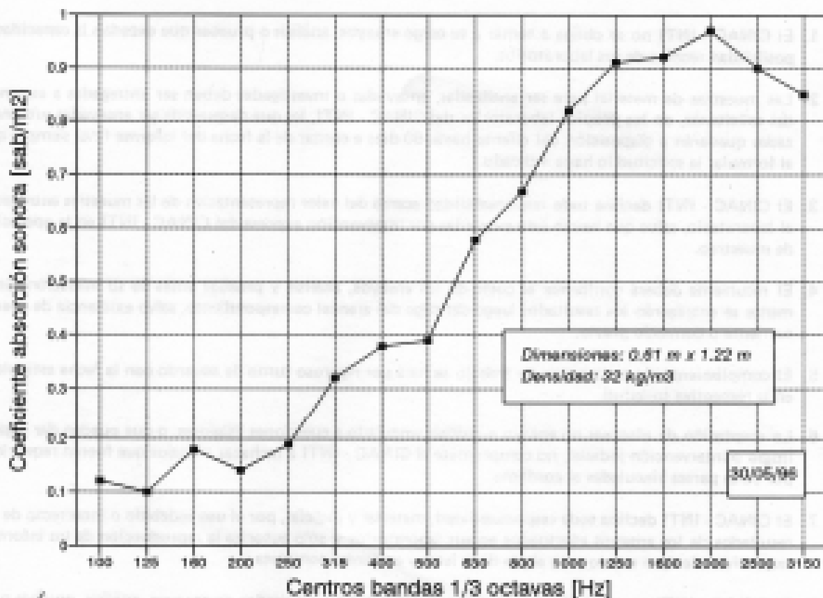
Figura 1: Placas FONAC PRO, e: 35 mm Laboratorio CINAC-INTI, norma IRAM 4065
