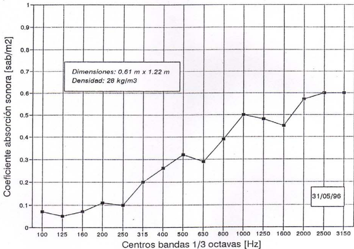
Figura 1: Placas FONAC ECO, e: 20 mm Laboratorio CINAC-INTI, norma IRAM 4065
