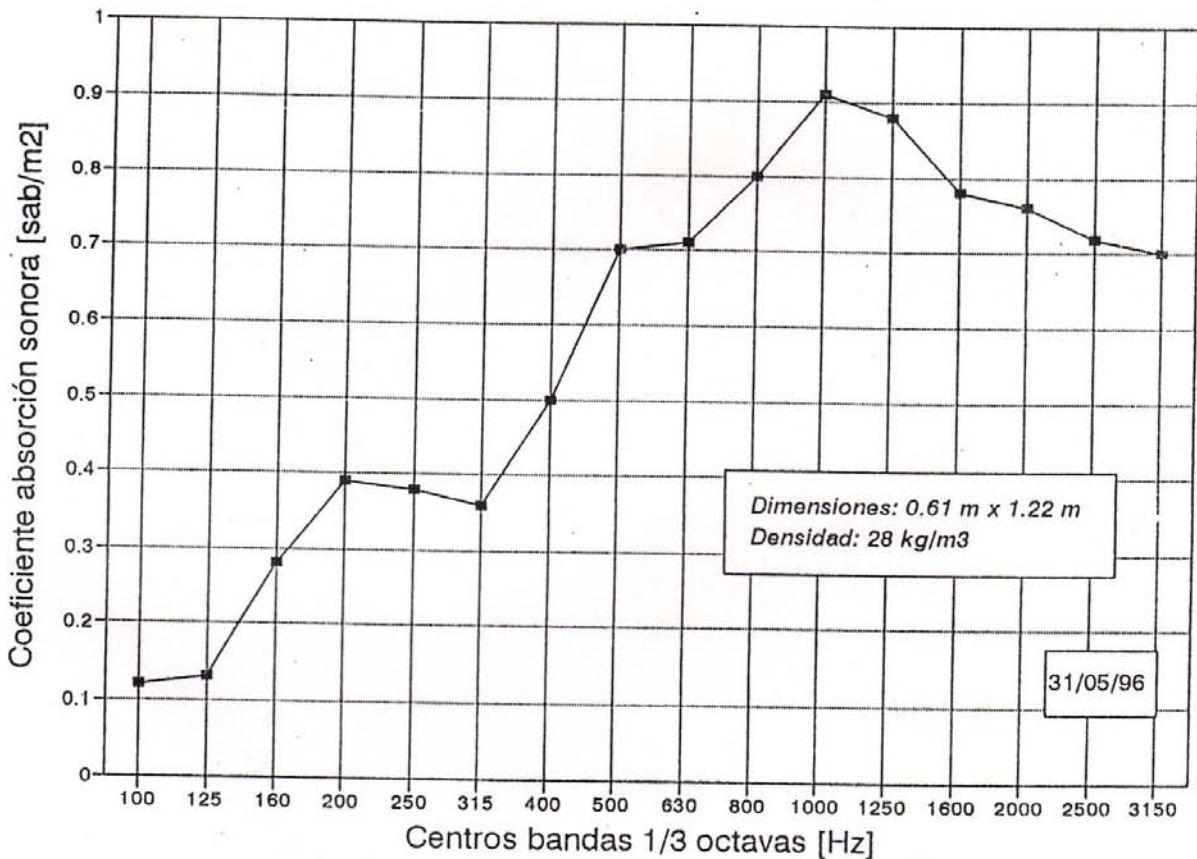
Figura 1: Placas FONAC ECO, e: 50 mm Laboratorio CINAC-INTI, norma IRAM 4065
