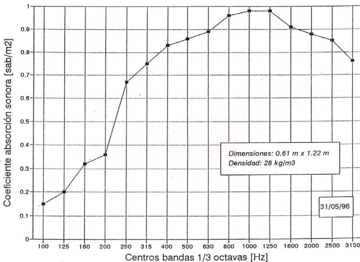
Figura 1: Placas FONAC ECO, e: 75 mm Laboratorio CINAC-INTI, norma IRAM 4065
