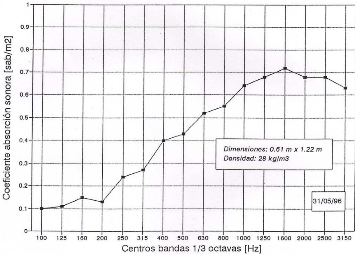
Figura 1: Placas FONAC ECO, e: 35 mm Laboratorio CINAC-INTI, norma IRAM 4065
